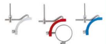
3-Stellungskampf Schnellwechselsystem (1 Glashalter, 3 Wechselsysteme) 3-Positions fast change system (1 glass holder, 3 change systems) 15
